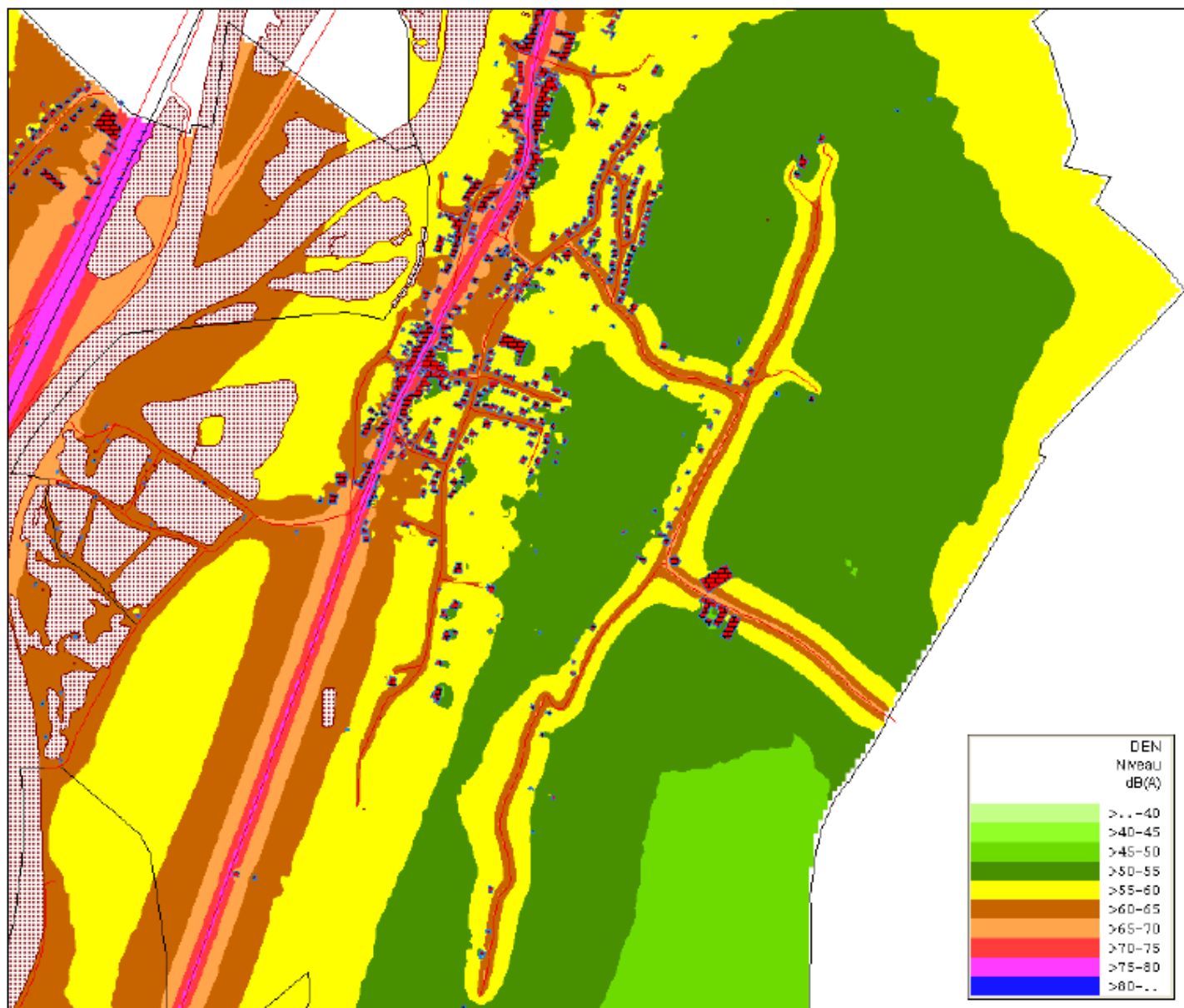
Carte de type A – Tout Bruit – Jouy-aux-Arches 1/2 – Lden – Echelle 1/10000
