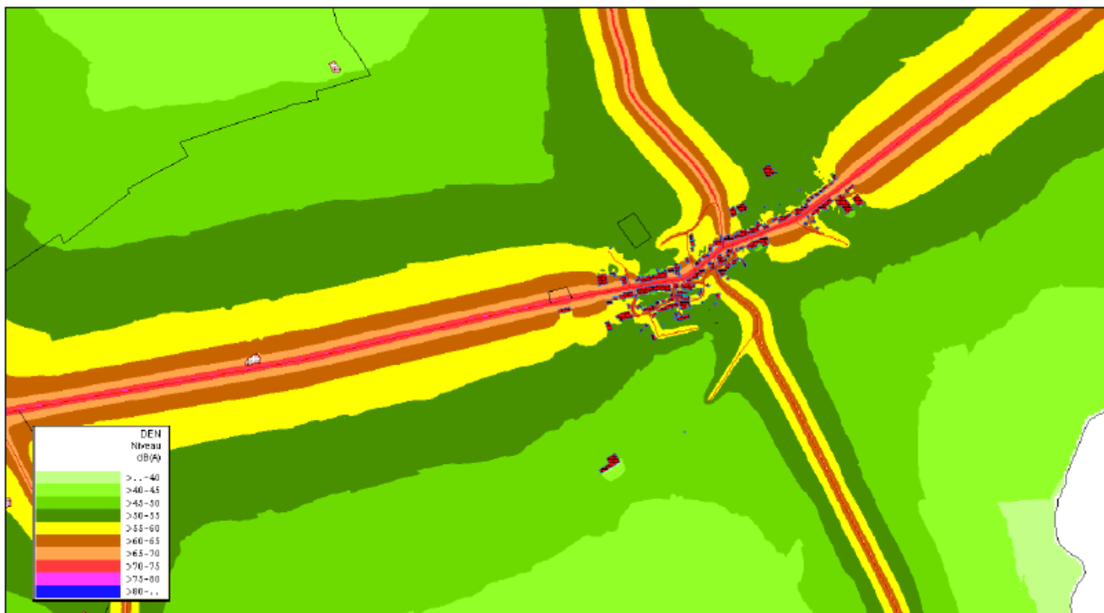
Carte de type A – Bruit routier – Rezonville – Lden – Echelle 1/10000
